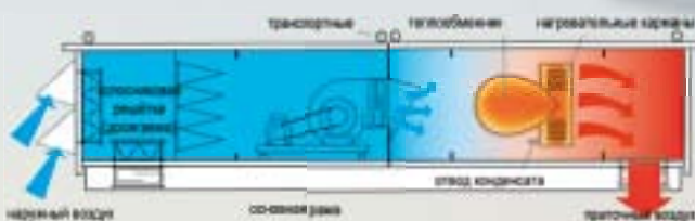
Функциональная схема
